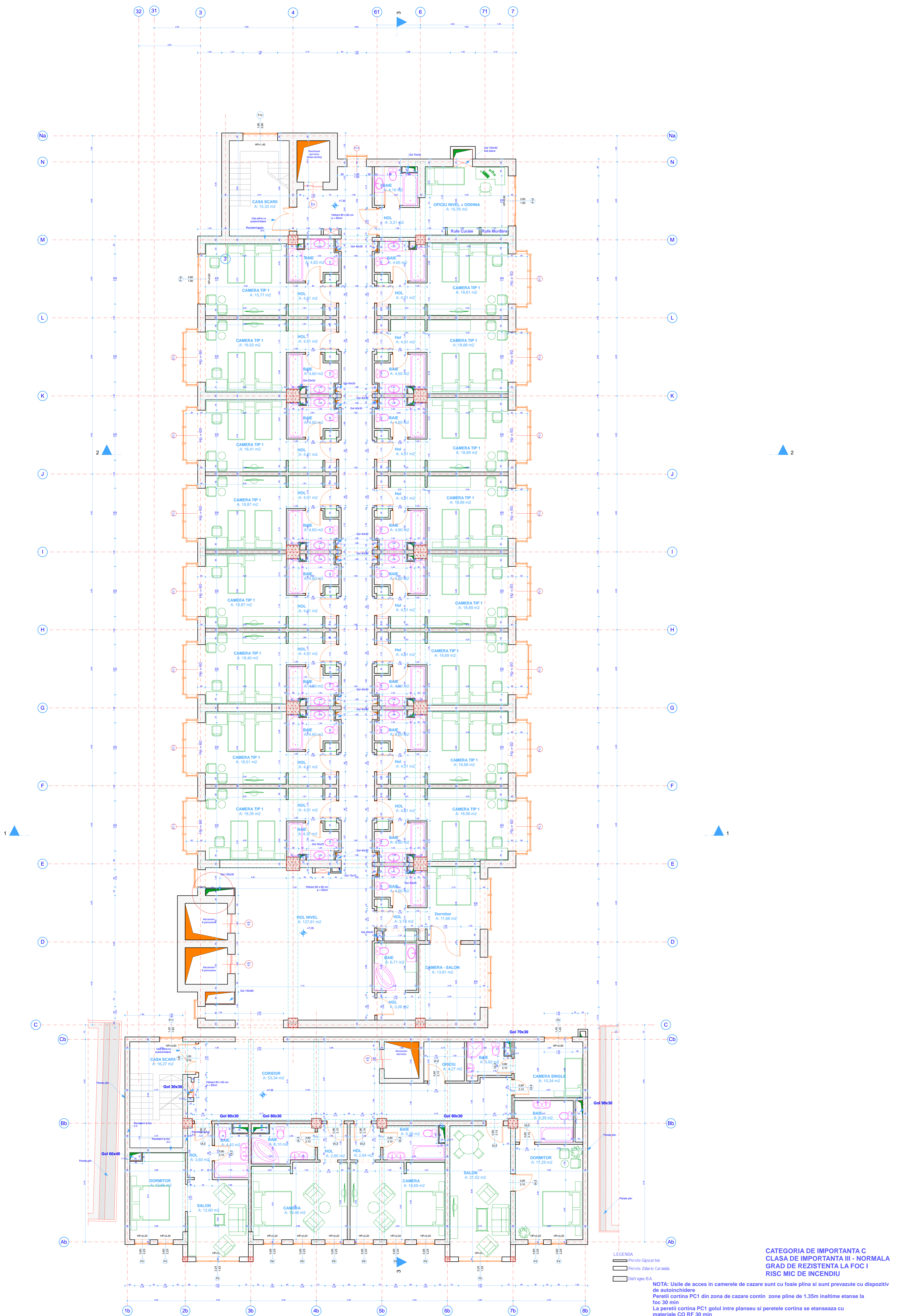
PLAN ETAJ 2-5
