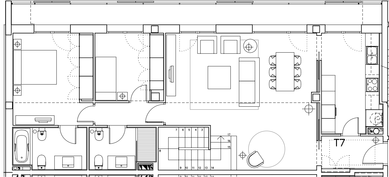
PLANTA ACCÉS HABITATGE – NIVELL 4
